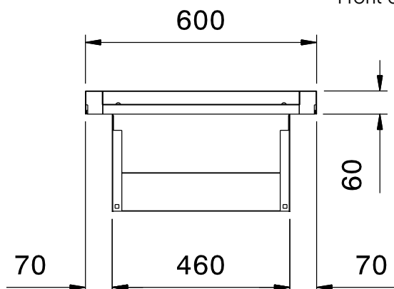
Front aanzicht
